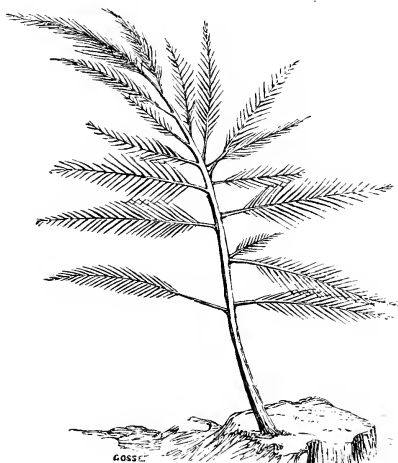
BRYOPSIS PLUMOSA.
